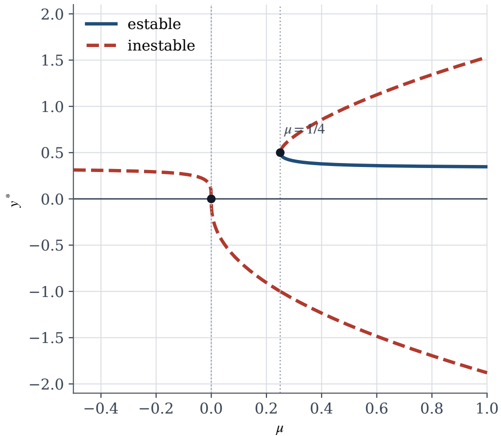
Equilibrios de y^3 - 3\mu y + \mu = 0
